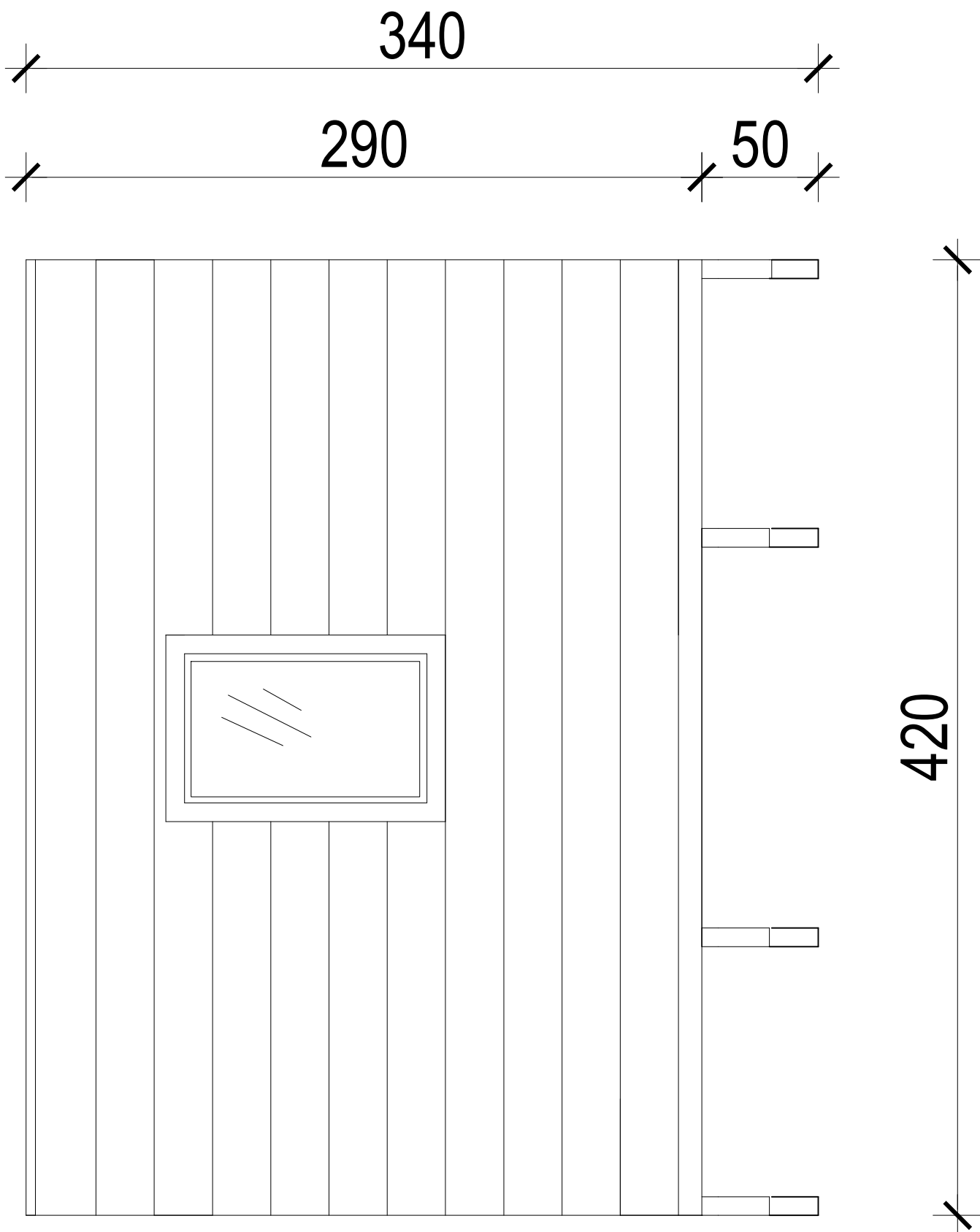
FASADA — BOČNO
